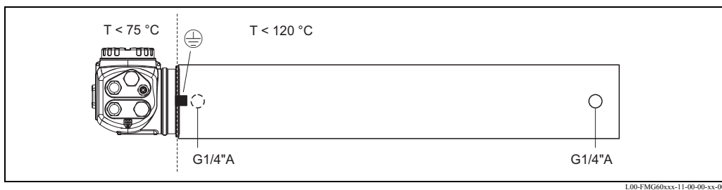
Подключение рубашки водяного охлаждения
