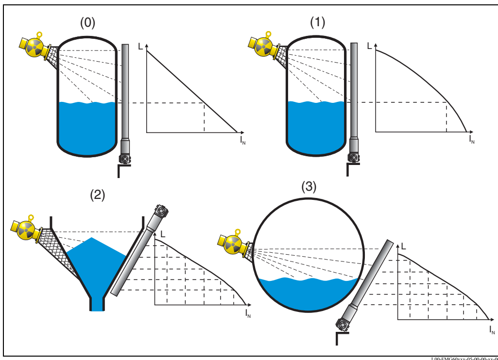
Режимы линеаризации при измерении уровня: (0): Линейный; (1): Стандартный; (2), (3): Заданная пользователем таблица линеаризации; I_N : Частота импульсов (имп/с); L: Уровень наполнения (%)
